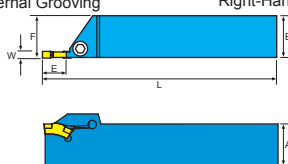
本圖所示為右手刀 (R) Right-Hand Show
