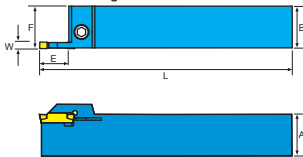
外徑切斷刀架 External Grooving
