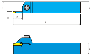
外徑切斷刀架 External Grooving
