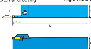
本圖所示為右手刀 (R) Right-Hand Show
