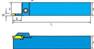
外徑切斷刀架系列 Tool Holders for External Deep Turning
